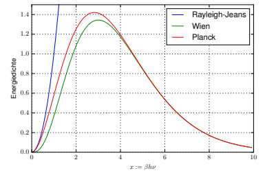
Strahlungsgesetze von Rayleigh-Jeans, Wien und Planck
