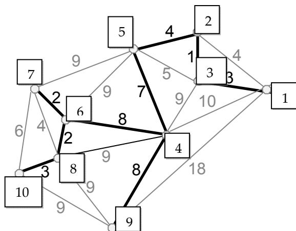
Ein minimaler Spannbaum
