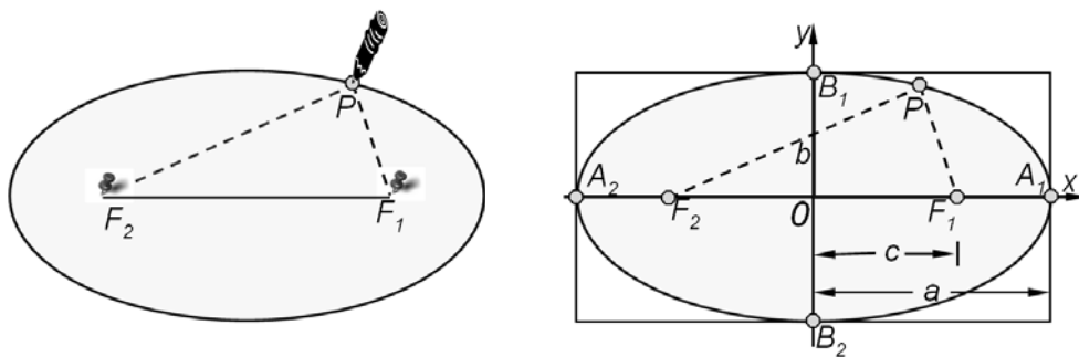
Ellipse: Konstruktionsverfahren; Scheitel und Achsen
