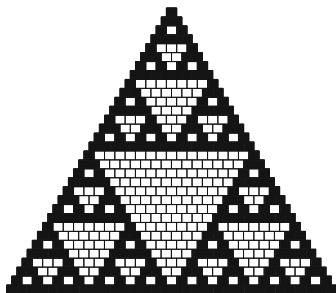
Bild 1.1 Pascalsches Dreieck modulo 2
